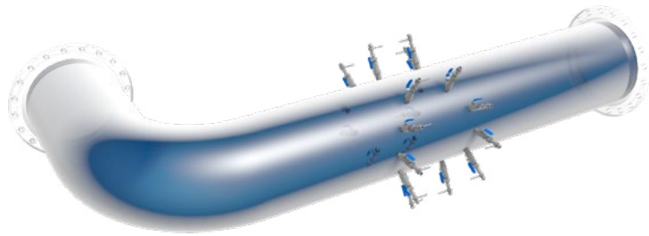
Ductus Installation nach einem 90°-Bogen
